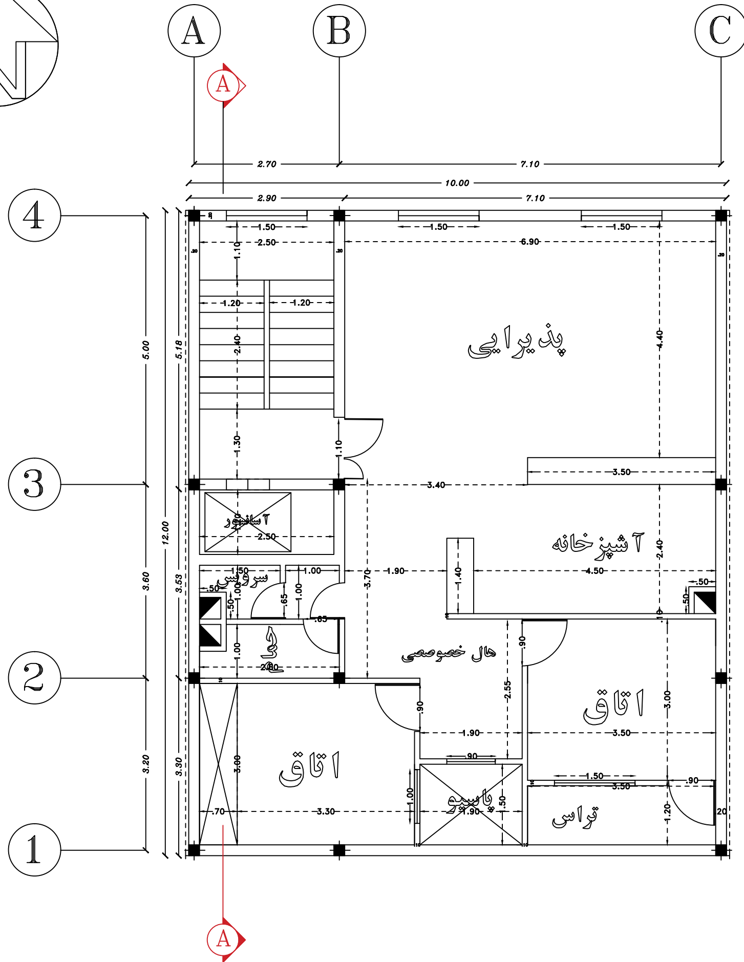
پلان تپ طبقات - اندازه گذاری
